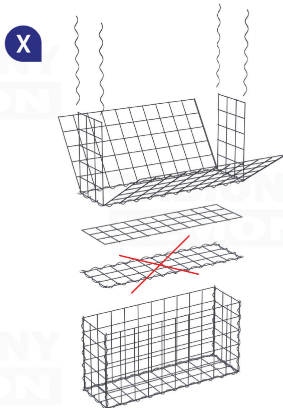
PRÍKLAD MONTÁŽE GABIÓNOVÝCH KOŠOV UKLADANÝCH NA SEBA
